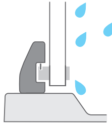
Rám v spodnej časti kúta: 10°, Pivot, Blix Slim, Blix, Supernova
