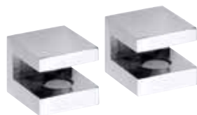
■ Držiak na poličku, pár Glass shelf holder – without glass, pair 20 x 20 x 25 mm ≠ 6 až 8 mm 102202112 bez DPH s DPH 11,0 € 13,1 €
